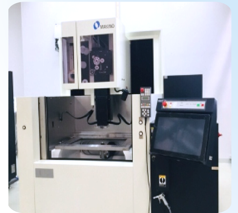
Makino U6 WEDM
